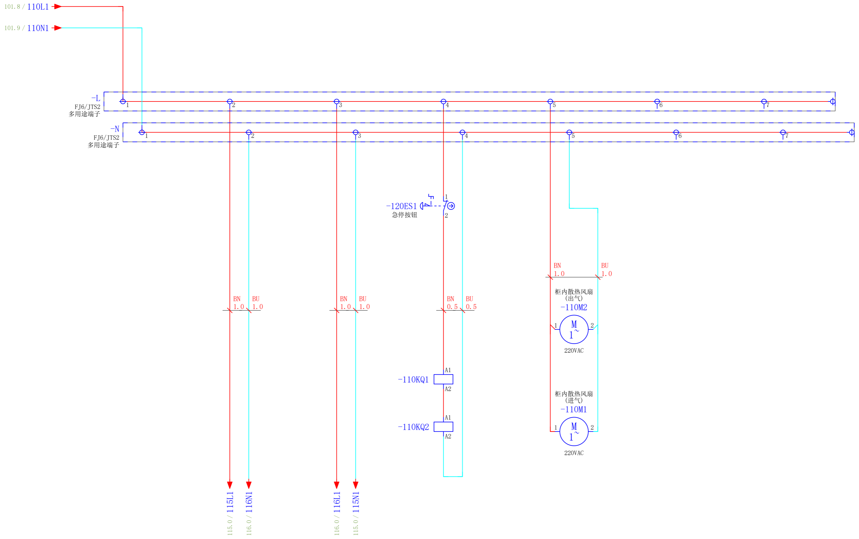
板卡/伺服抱闸开关电源 220VAC供电
